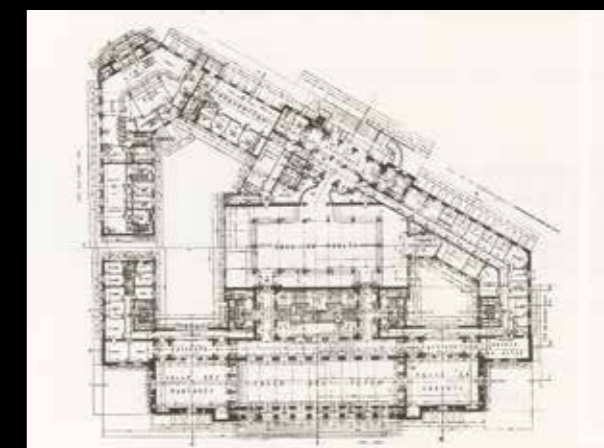
Plans du rez-de-chaussée
