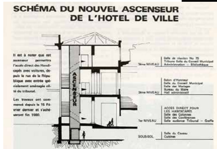
Schéma du nouvel ascenseur de l'Hôtel de Ville, bulletin municipal de juin 1980, 1PER/1, AMP.
